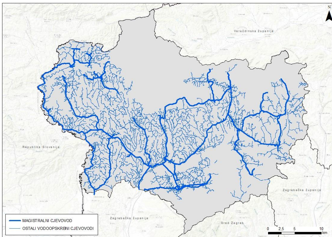
Slika 30. Kartografski prikaz vodoopskrbne mreže na području Krapinsko-zagorske županije u nadležnosti Zagorskog vodovoda d.o.o.
